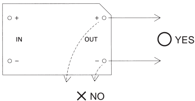
Fig.5.1 Pattern wiring
